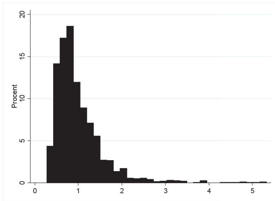
Figur 2: Vægtens fordeling (størrelsen af weight_1)
